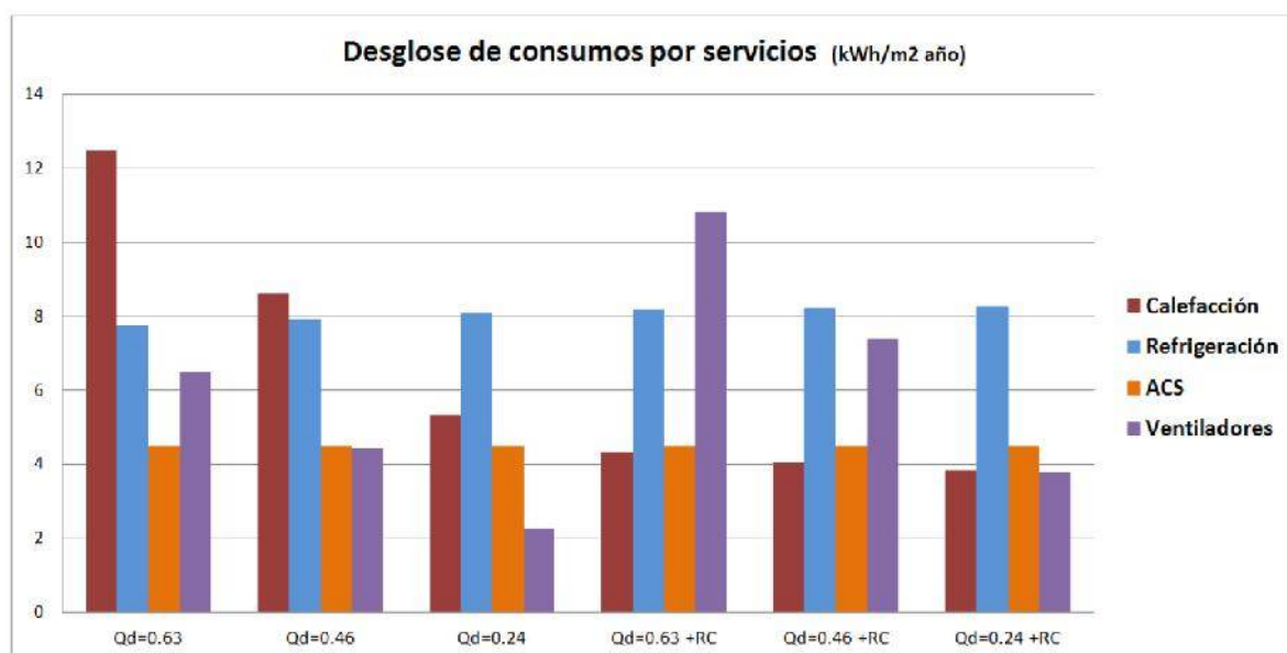
Fig.13. Estudio de consumos por servicios en un edificio plurifamiliar en Madrid en función de diferentes caudales de ventilación de diseño ( Q_d ) y de la utilización o no de recuperadores de calor (RC) con rendimientos del 80% y SFP de ventiladores de 2,5kPa
