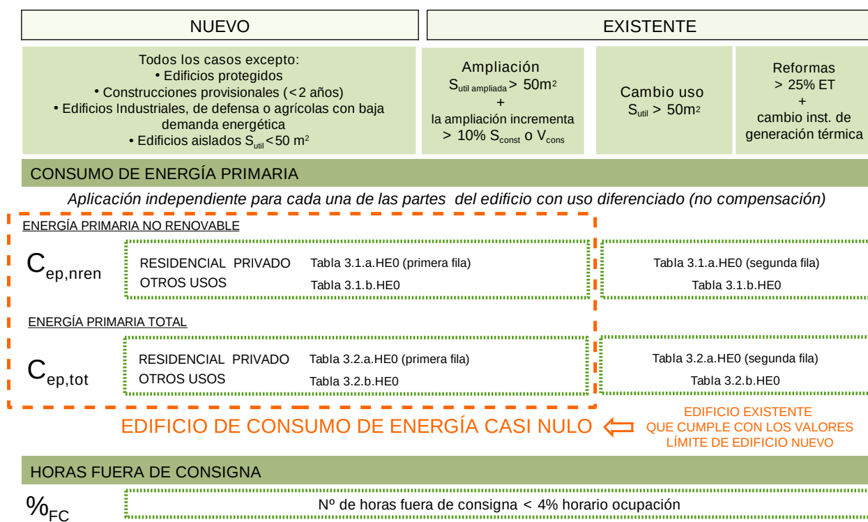
Fig.4. Esquema aplicación HE0
